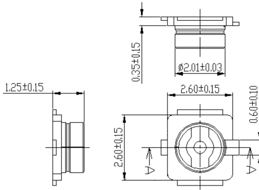
图 4-28 IPEX 座子尺寸
