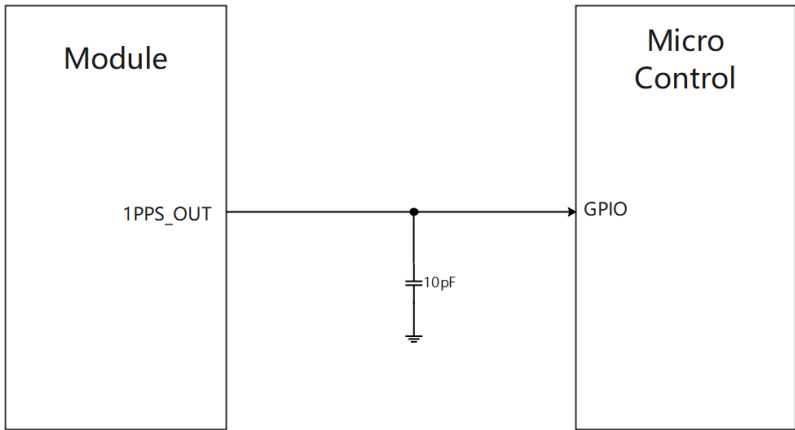
图 4-25 1PPS_OUT 接口推荐电路
