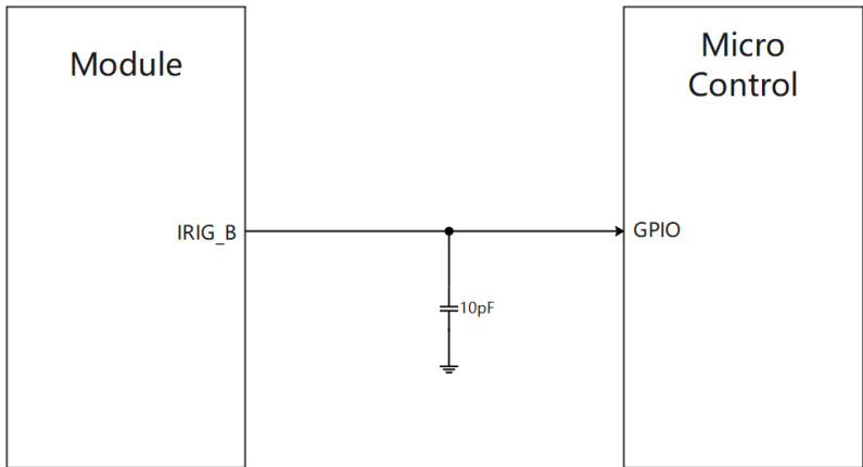
图 4-24 IRIG_B 接口推荐电路
