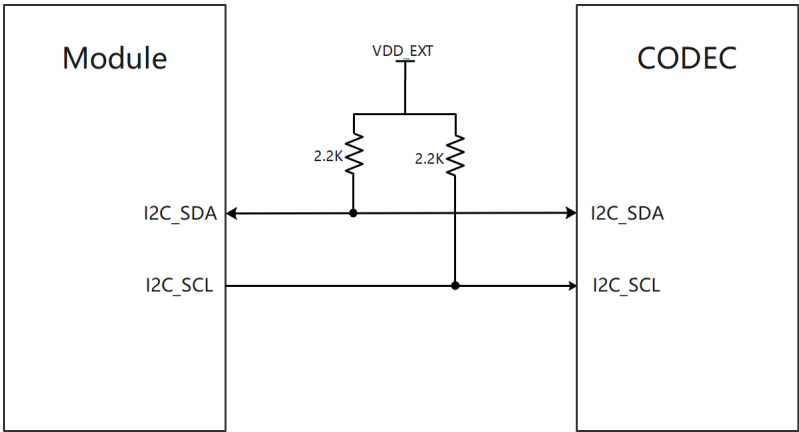
图 4-23 I2C 接口推荐电路
