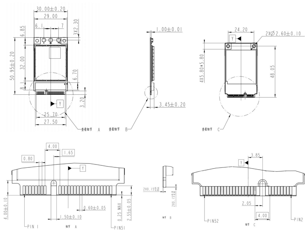
图 7-1 模块结构图(单位：mm)
