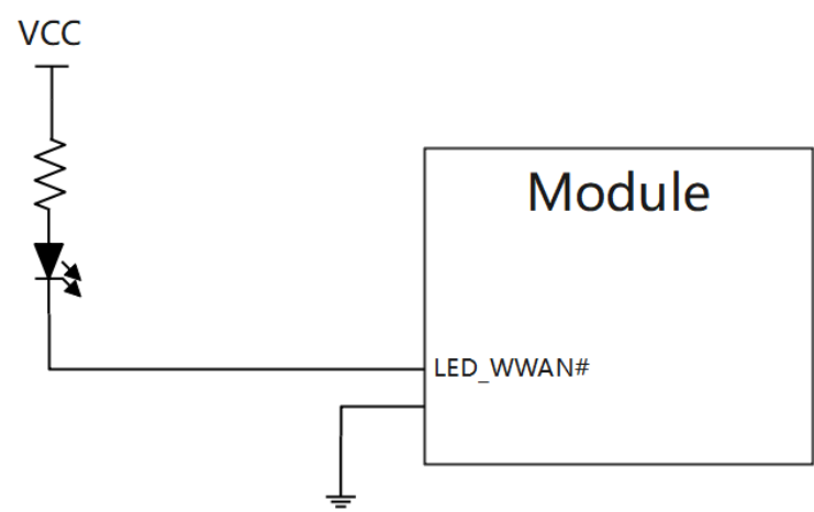
图 4-26 LED 推荐设计电路
