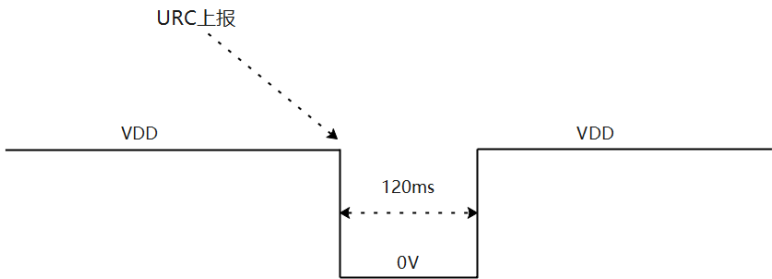
图 4-6 WAKE# 逻辑
