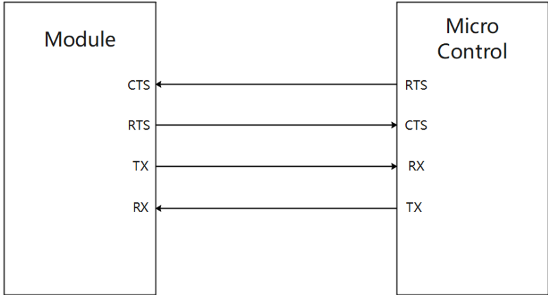
图 4-19 四线 UART 推荐电路
