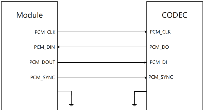
图 4-22 PCM 接口推荐电路
