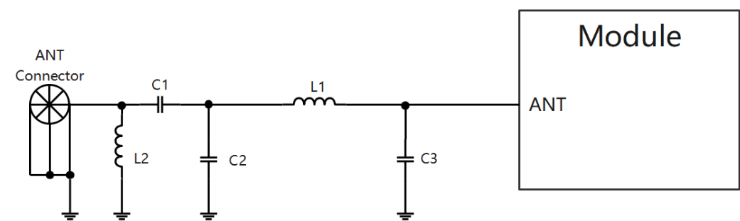
图 4-27 天线走线推荐电路
