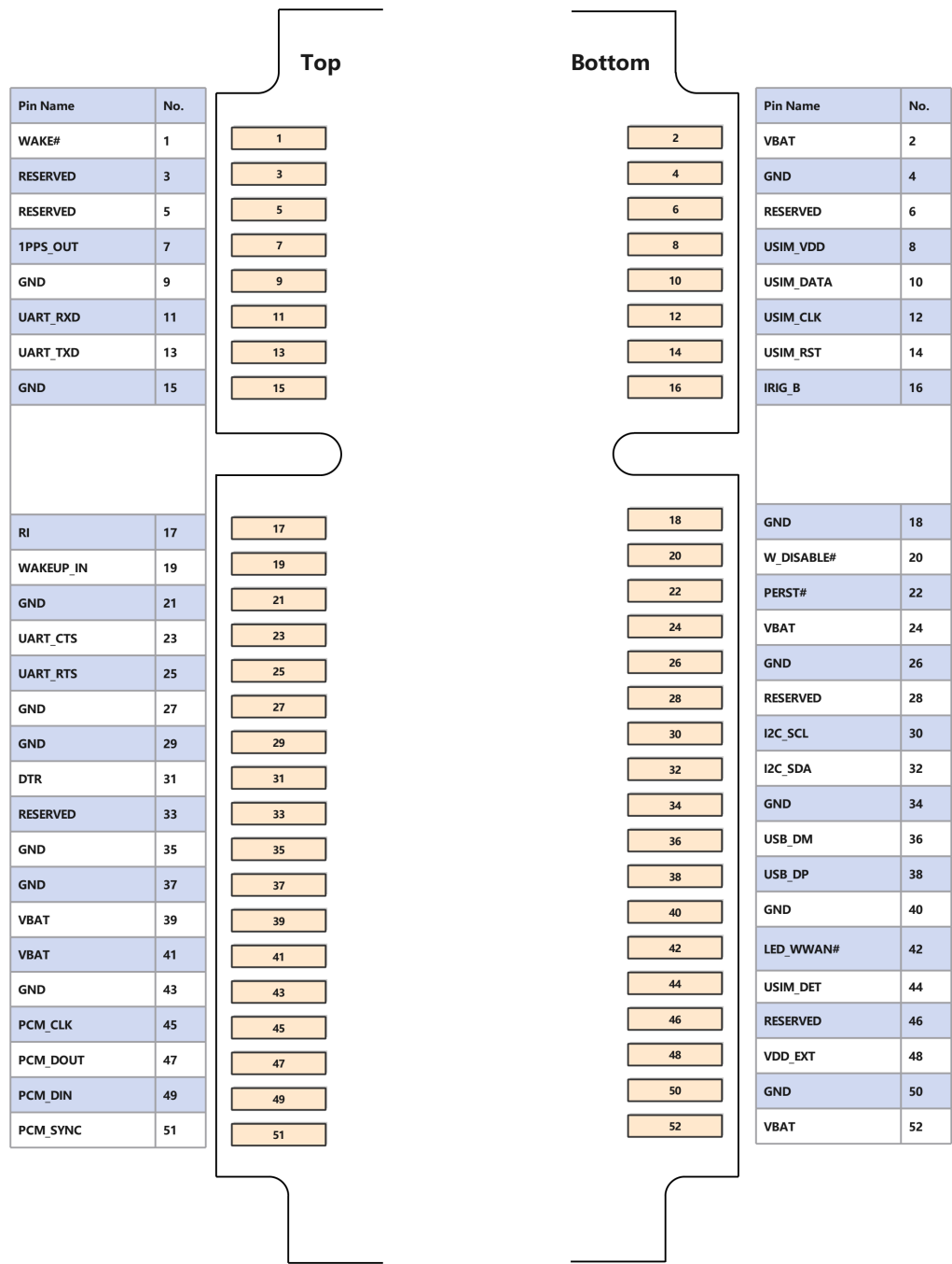
图 4-2 模块引脚分布图
