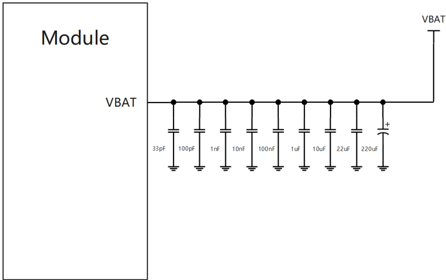
图 4-3 VBAT 引脚参考电路
