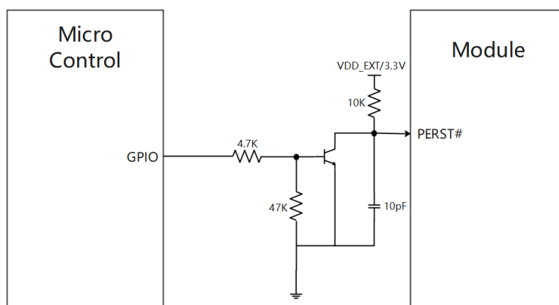
图 4-14 PERST#引脚推荐电路 2
