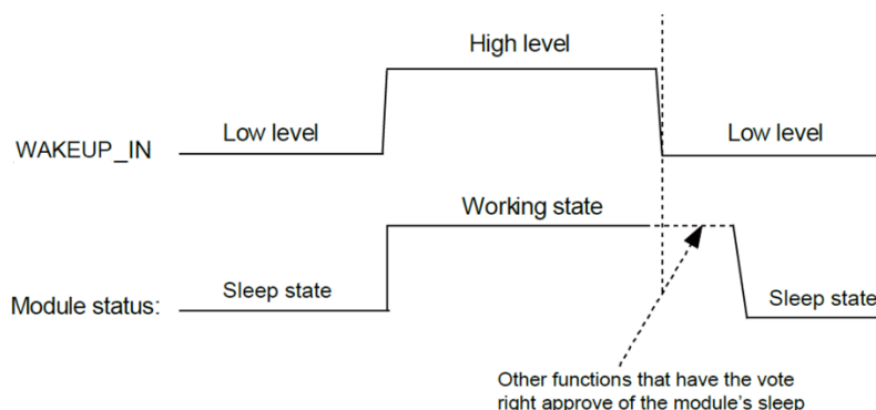
图 4-10 WAKEUP_IN 引脚时序
