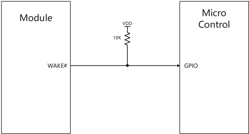
图 4-6 WAKE# 逻辑
