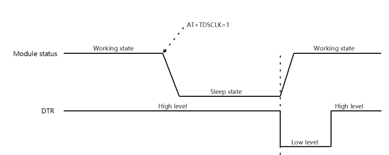
图 4-15 采用 AT 指令+DTR 组合进行休眠唤醒逻辑及时序
