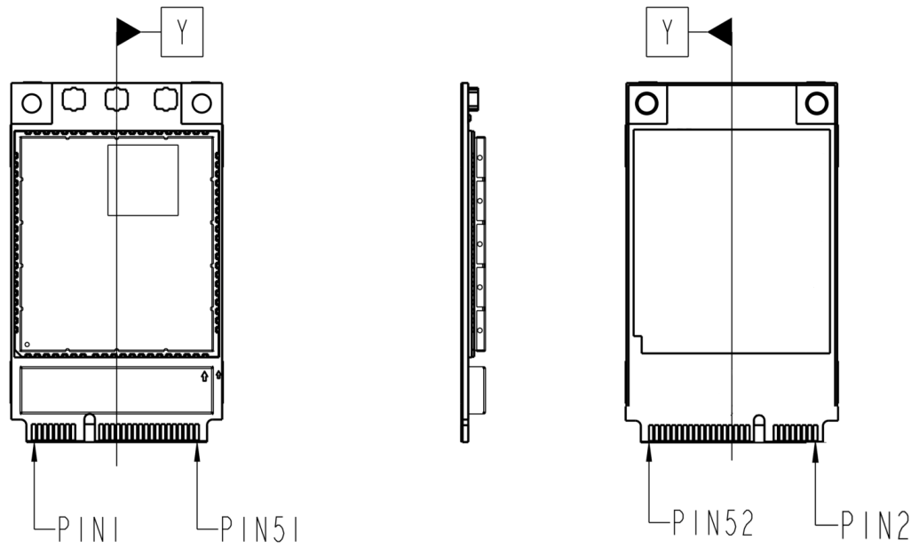
图 4-1 模块管脚顺序图
