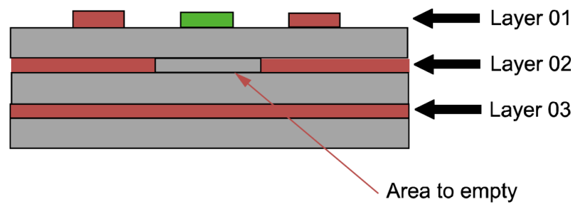
图 6-5 RF PAD 隔层参考示意图
