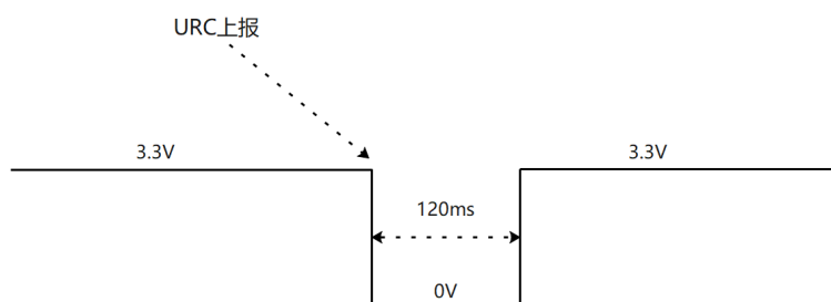
图 4-8 RI 逻辑
