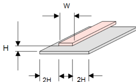
图 6-2 微带线
