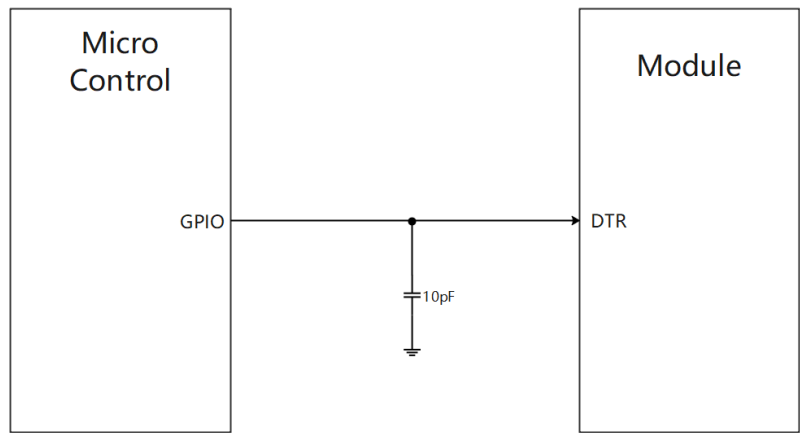
图 4-16 DTR 引脚推荐电路 1
