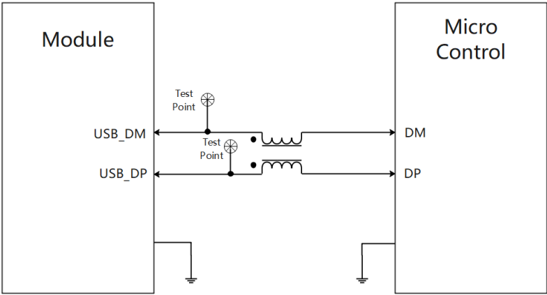
图 4-20 USB2.0 推荐电路
