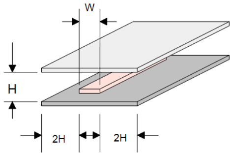
图 6-3 带状线
