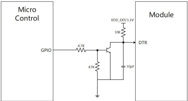
图 4-17 DTR 引脚推荐电路 2
