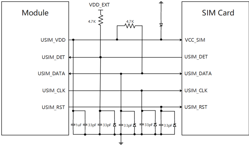
图 4-21 USIM 卡推荐电路
