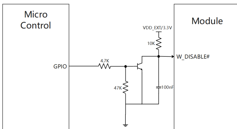
图 4-12 W_DISABLE#引脚推荐电路 2
